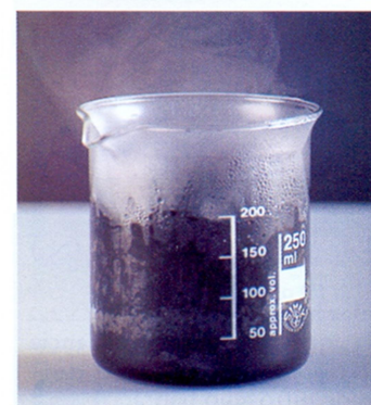
Reacción exotérmica.
