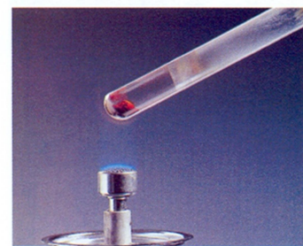
Reacción endotérmica.
